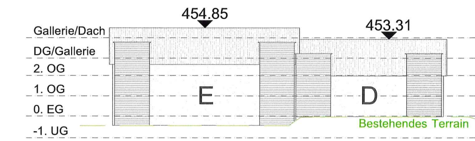
Südfassade Haus E/D
