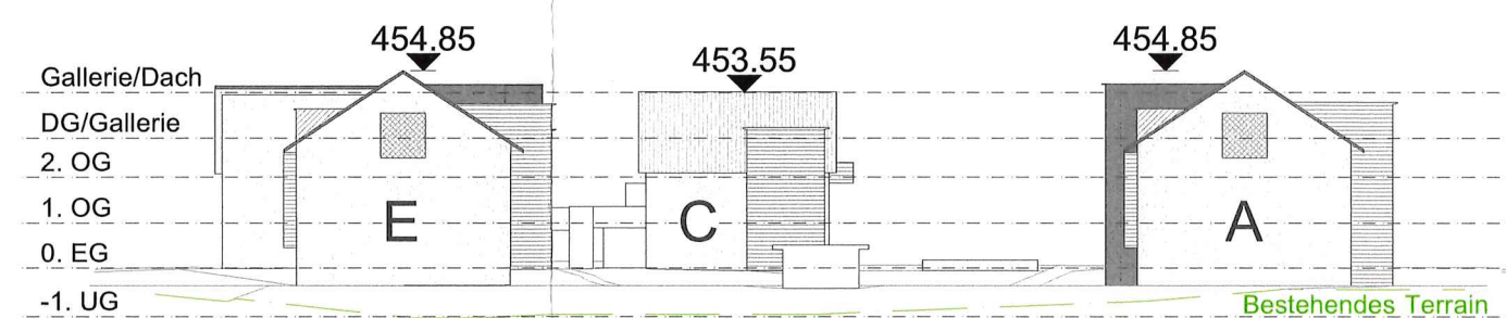
Westfassade Haus E/C/A
