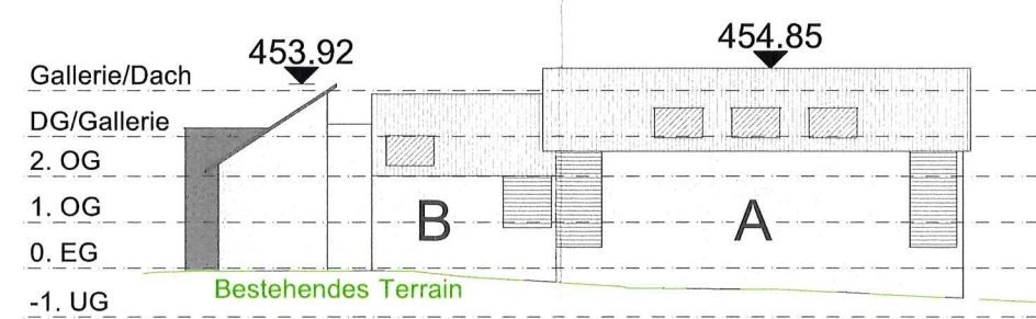
Nordfassade Haus B/A
