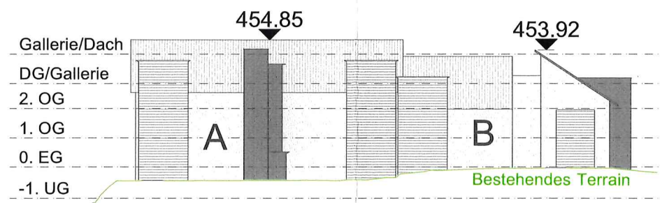
Südfassade Haus A/B
