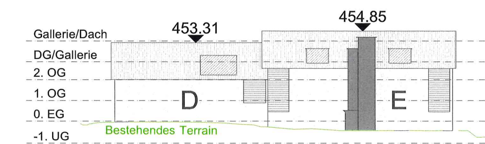
Nordfassade Haus D/E
