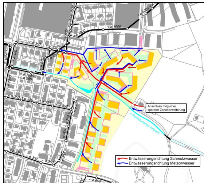
Konzeptionelle Entwässerung, Auszug aus GEP-Nachführung Lüssi Göbli
